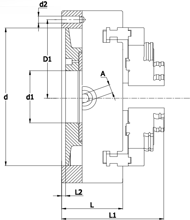
TEKNİK ÖLÇÜLER(mm ) / Technical Dimensions
